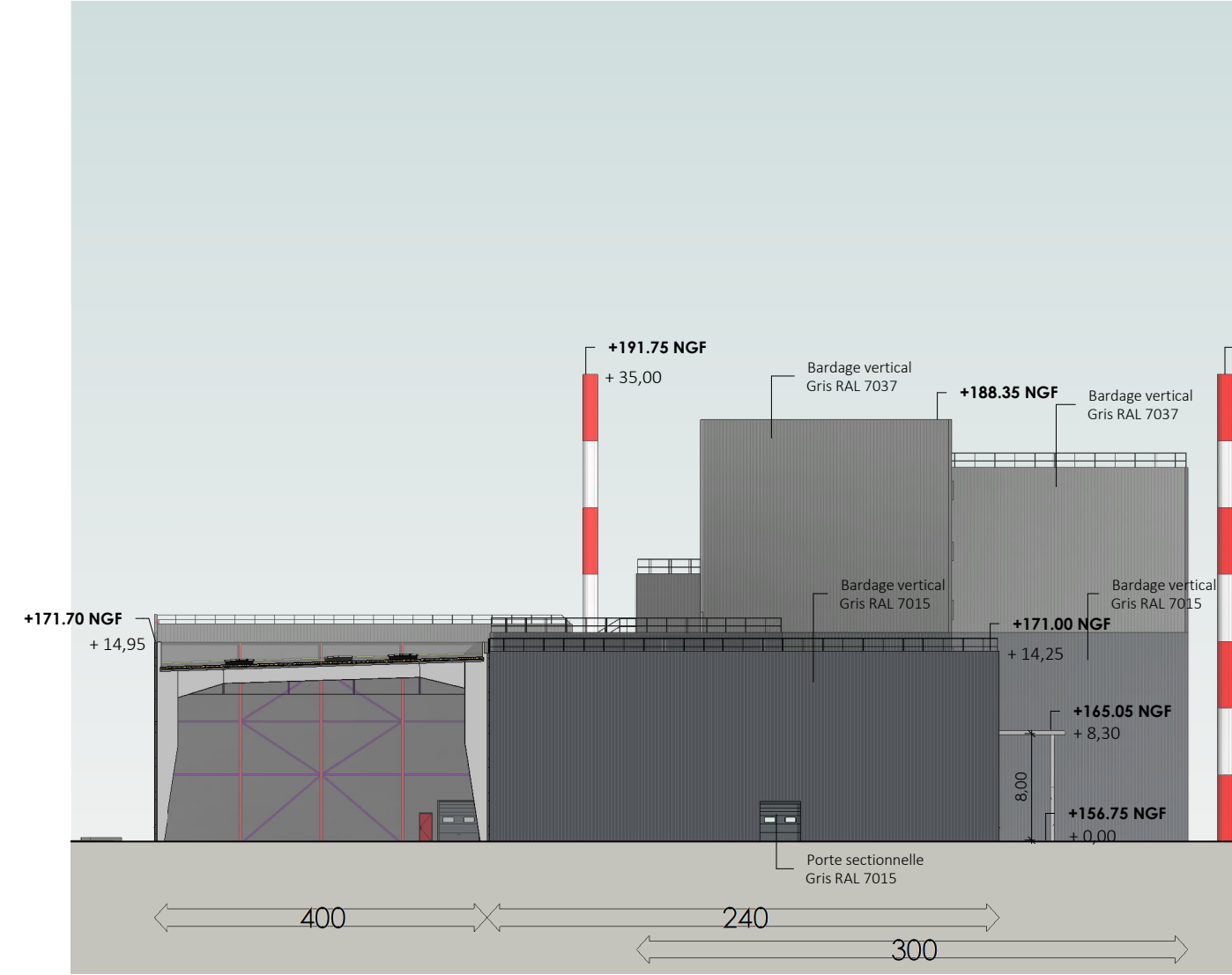
8 Façade Sud-B240 1:500
