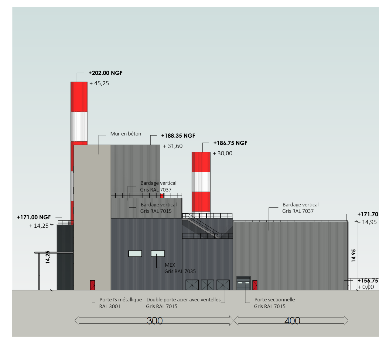
4 Façade Nord 1:500
