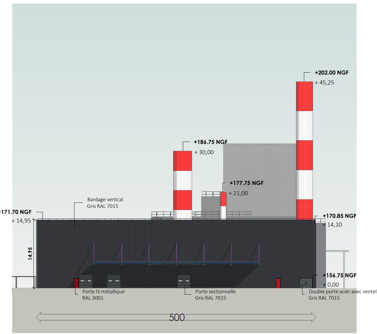
6 Façade Sud 1:500
