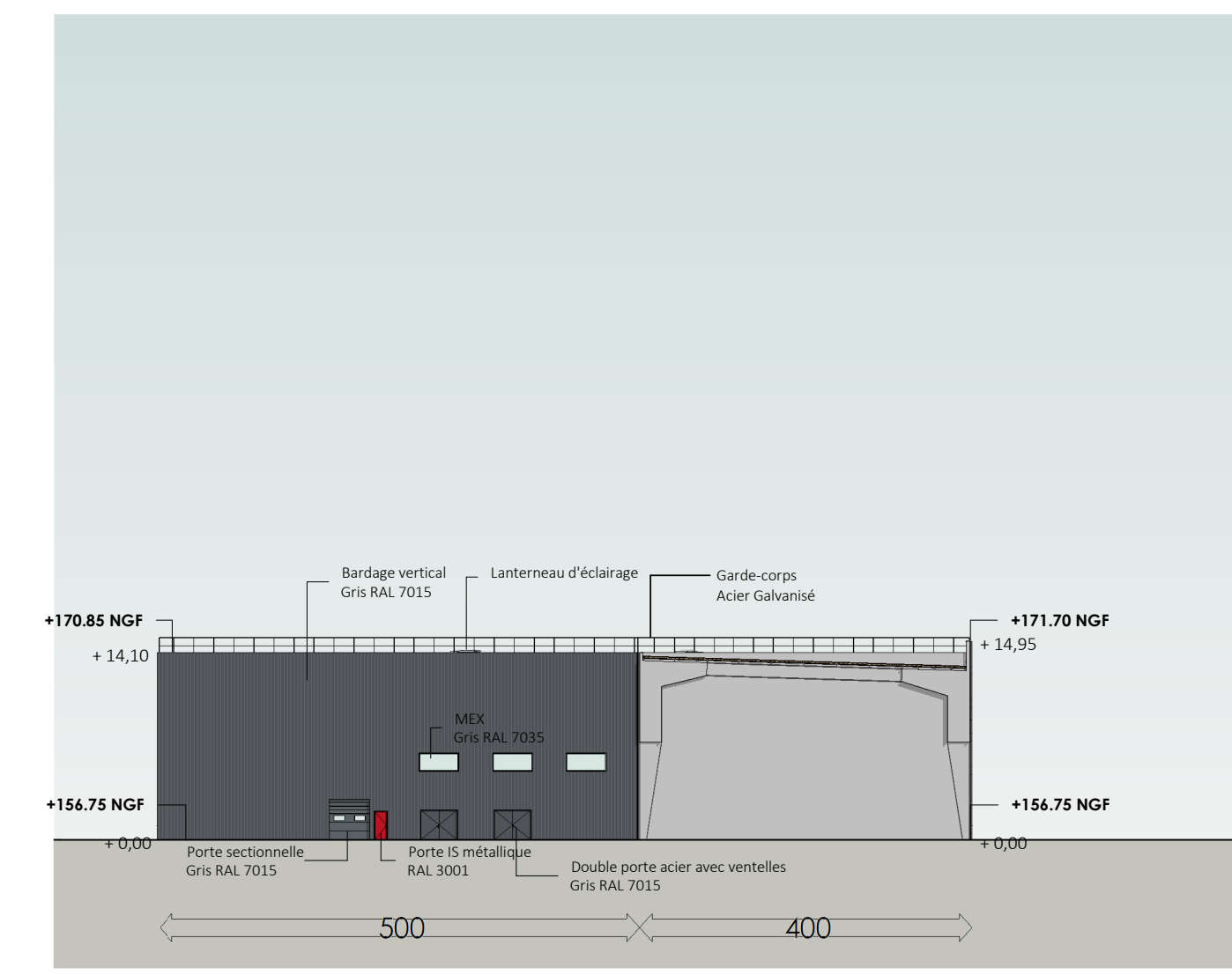
7 Façade Nord B400 1:500
